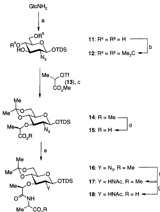
Scheme 2. Synthesis of muramic acid derivative 18 ; a) refs. 26,27; b) (MeO) 2 CMe 2 , p -TsOH (quant.); c) NaH, CH 2 Cl 2 (70–95%); d) LiOH, dioxane/MeOH (quant.); e) L-Ala-OMe·HCl, EEDQ NEt 3 , CH 2 Cl 2 (85%); f) H 2 S, Pyr/H 2 O; Ac 2 O, pyr (89%); g) LiOH, dioxane/MeOH (quant.)
